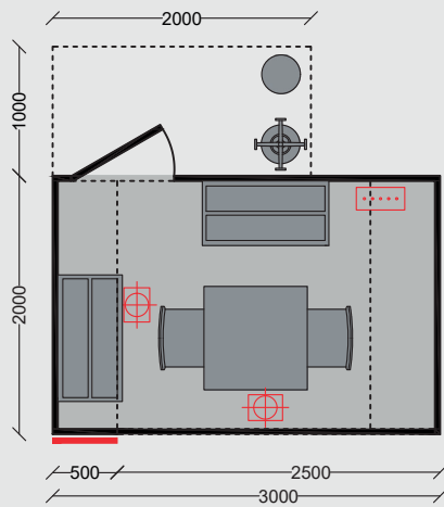
Ripostiglio esterno con apertura porta interna, posizionato su lato sinistro dello stand / External storage room with internal door opening, positioned on the left side of the stand
